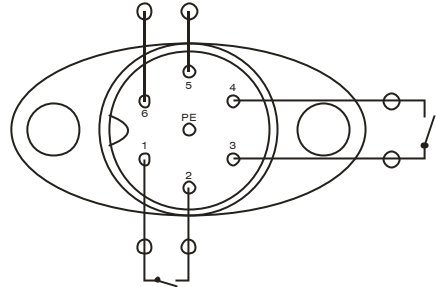
Figure 4: Affectation des contacts de la prise de Reset / cycle / moniteur
